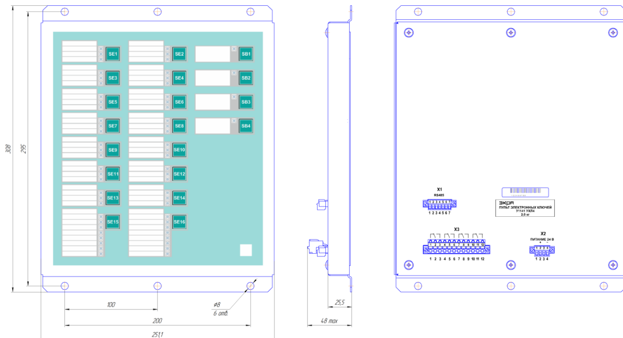
Рисунок 1 – Общий вид и габаритные размеры пульта электронных ключей У1141
